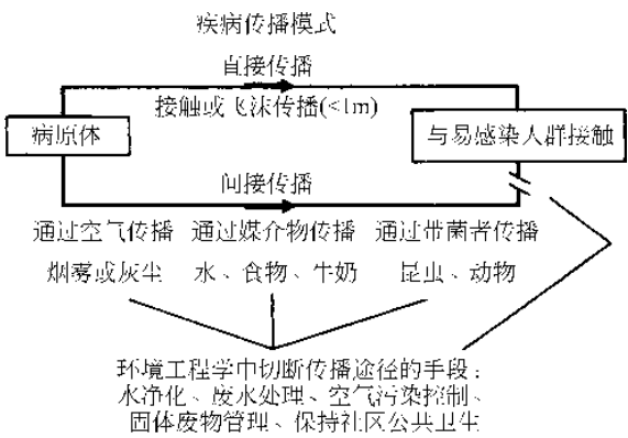
图 1.2 传染性疾病可以通过一些途径进行传播,应用现代环境技术可以控制许多传播途径。
