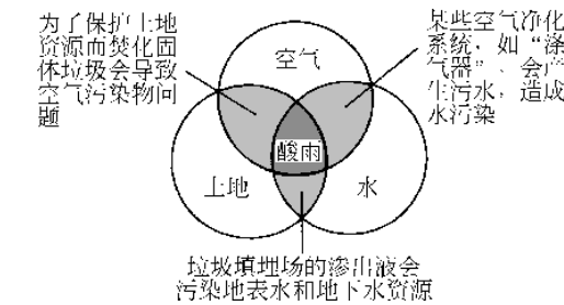
图 1.1 大部分空气、水和土壤的环境问题都是有联系的。例如,酸雨是空气污染所引起的,而酸雨会破坏水、陆地生态系统。
