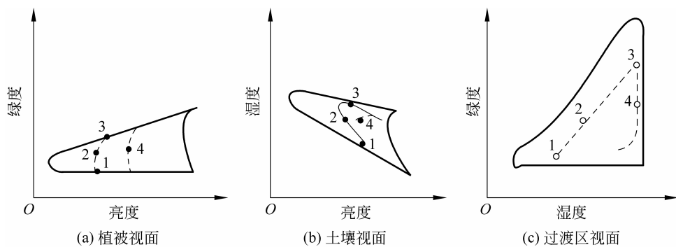
1. 裸土(种子破土前); 2. 生长; 3. 植被最大覆盖; 4. 衰老
