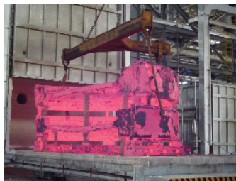
图 1-19 大型零件热处理
