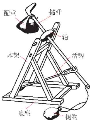
图 1-7 古代机械——元代回回炮
