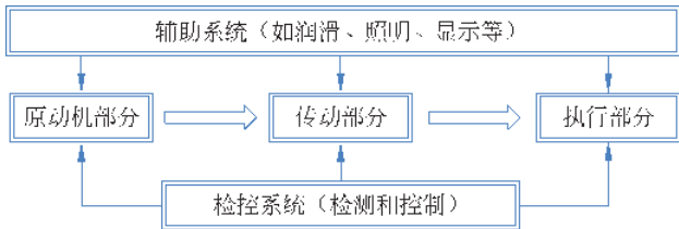
图 1-10 机器的组成
