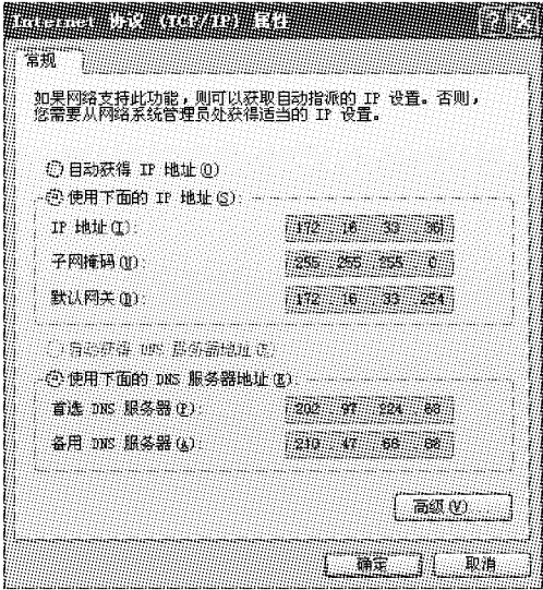
图 3-10 “Internet 协议(TCP/IP)属性”对话框
