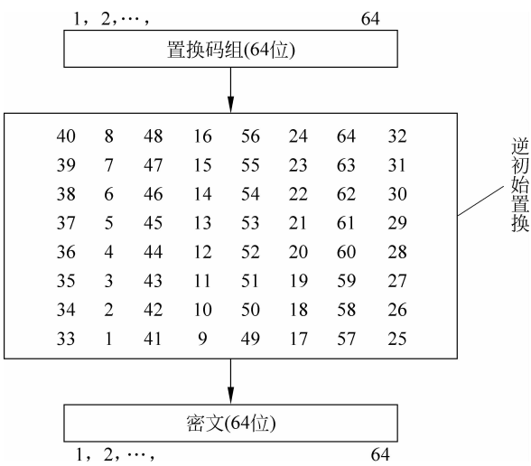
图 3-10 逆初始置换 IP^{-1}
