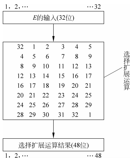
图 3-4 选择扩展运算 E
