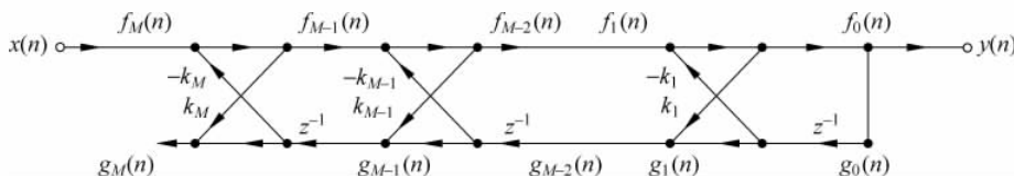
图 5.37 全极点 IIR 系统的格型结构
