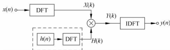
图 5.20 FIR 滤波器的快速卷积结构
