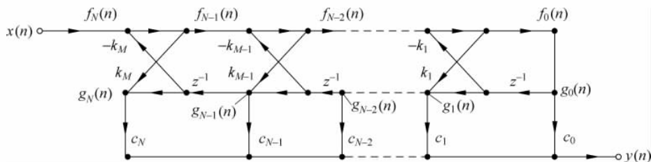
图 5.39 零-极点型 IIR 系统的格型结构
