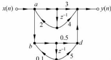
图 5.28 滤波器结构
