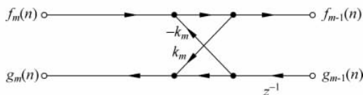
图 5.36 全极点 IIR 系统格型结构的基本单元
