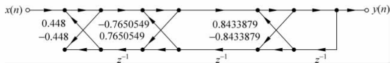
图 5.38 例 5.8 的全极点型 IIR 滤波器的格型结构
