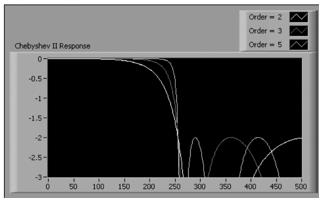
图 5-6 反切比雪夫低通滤波器的幅频特性曲线
