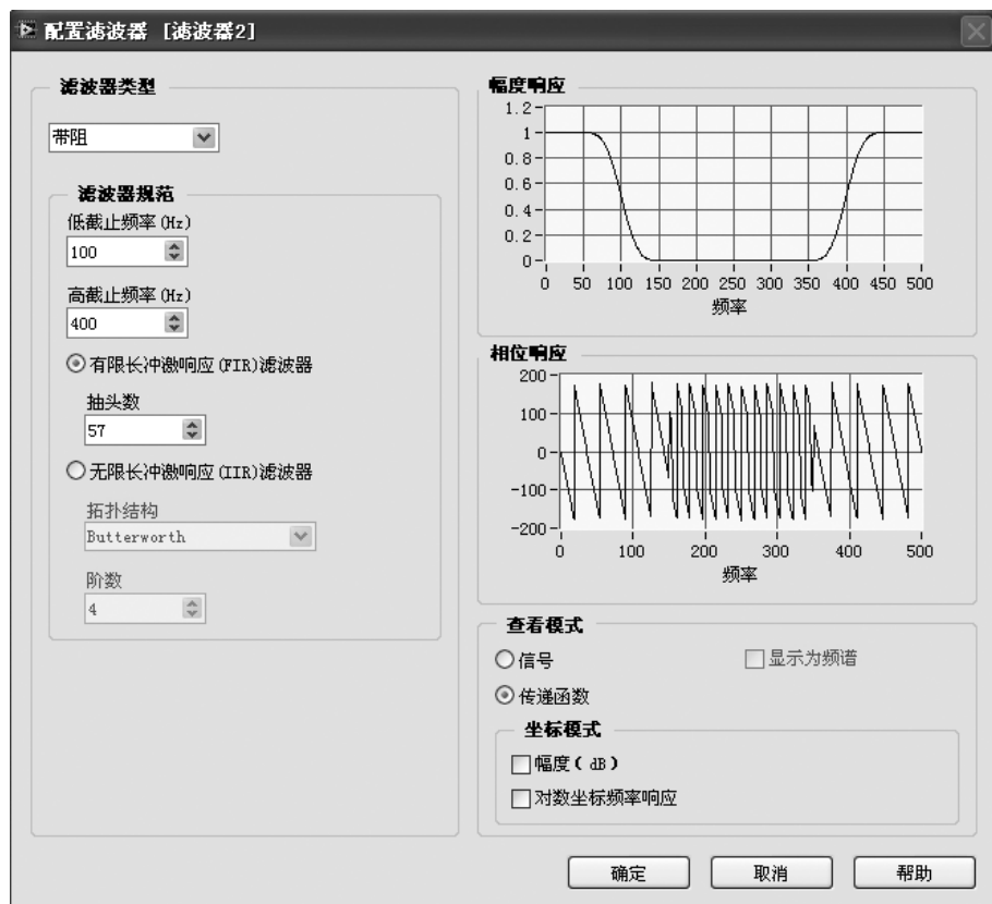
图 5-13 带阻 FIR 滤波器配置对话框
