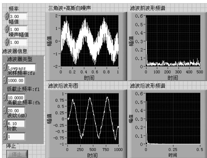
图 5-33 Chebyshev 滤波器 VI 对混有均匀白噪声的三角波信号进行滤波
