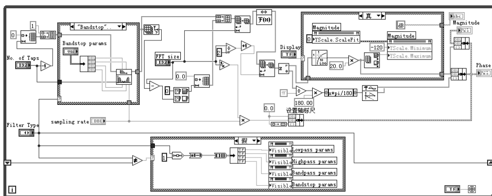
图 5-28 使用基于 Parks-McClellan 算法的等波纹优化滤波器设计实现 FIR 滤波器
