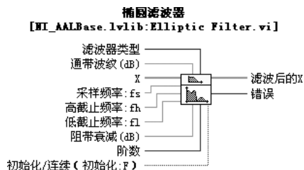
图 5-36 椭圆滤波器 VI 的图标和端口
