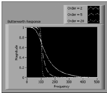
图 5-4 巴特沃斯低通滤波器的幅频特性曲线
