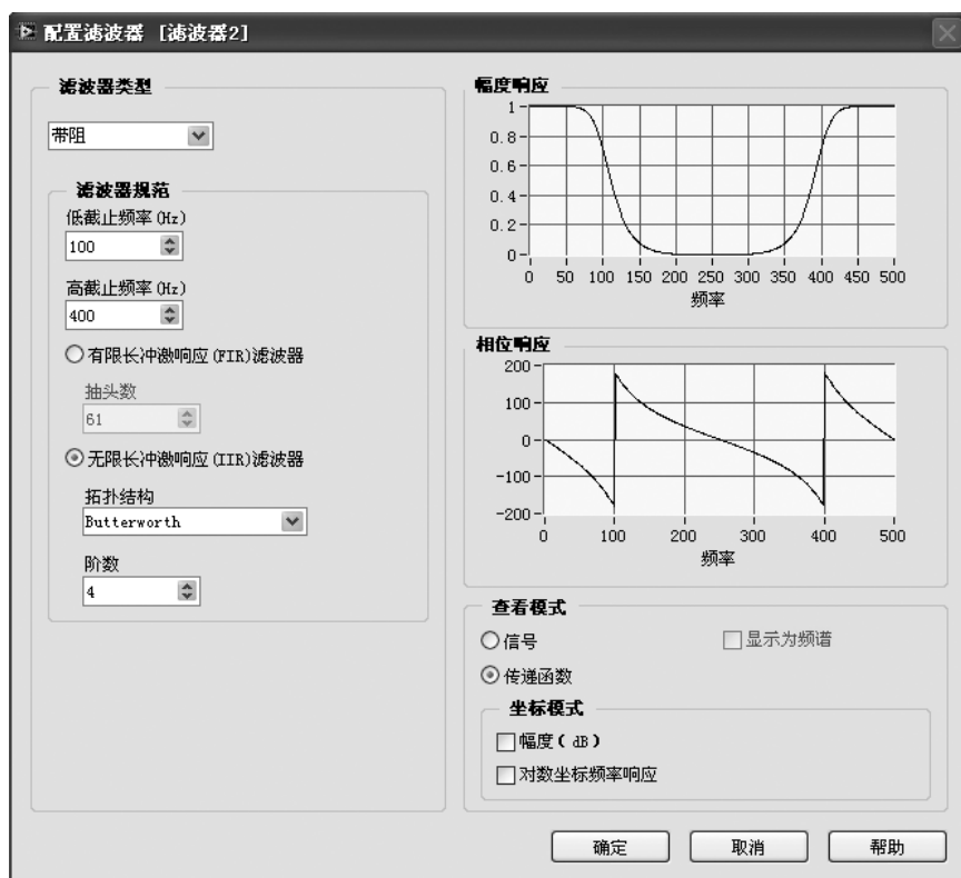
图 5-12 巴特沃斯带阻 IIR 滤波器配置对话框
