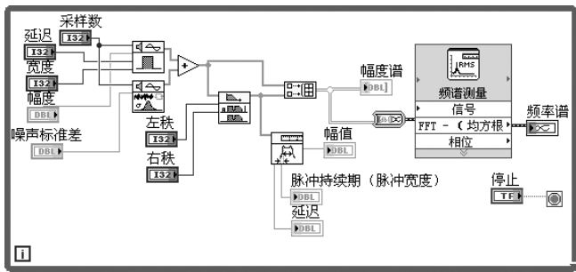
图 5-43 使用中值滤波器 VI 对混有高斯白噪声的脉冲信号进行滤波 (续)
