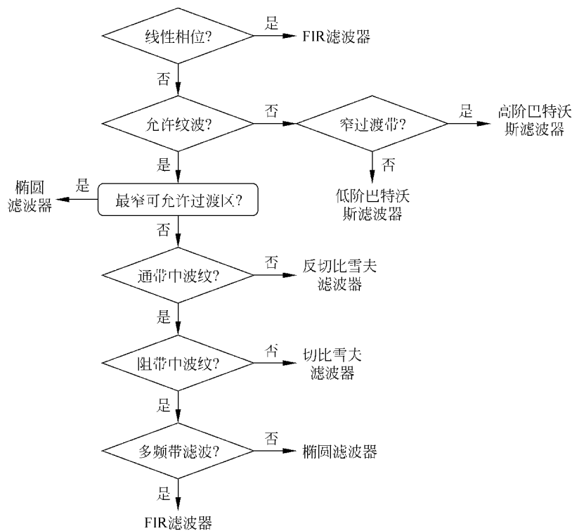
图 5-10 滤波器选择向导流程图
