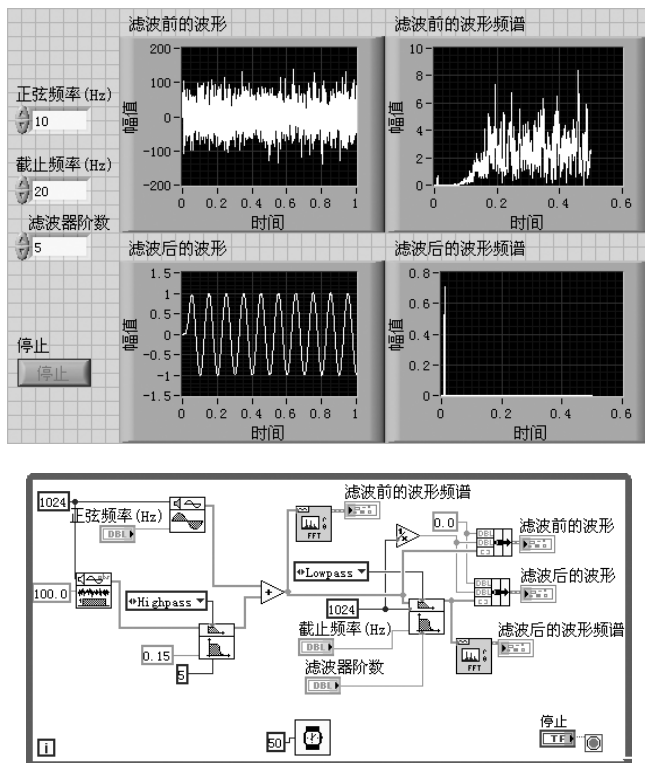
图 5-31 使用巴特沃斯滤波器提取正弦波形并对其进行频谱分析显示
