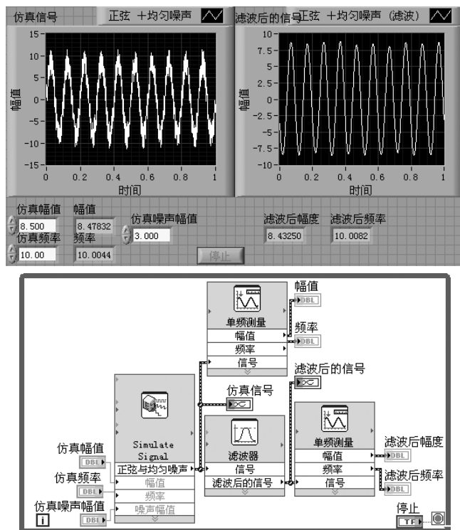
图 5-15 Express 滤波器
