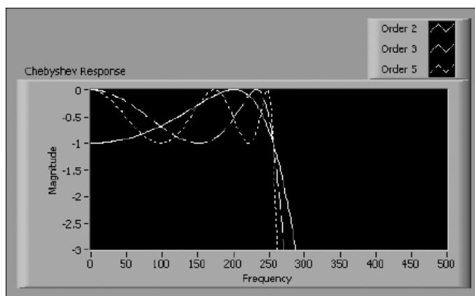
图 5-5 切比雪夫低通滤波器的幅频特性曲线
