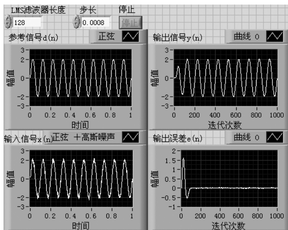
图 5-49 基于 LMS 算法设计实现自适应滤波器
