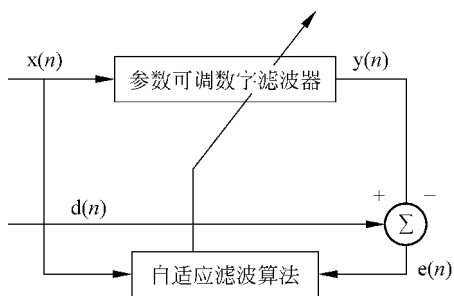
图 5-44 自适应滤波器结构
