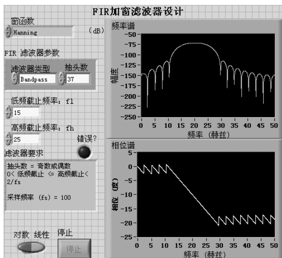
图 5-27 FIR 加窗滤波器设计
