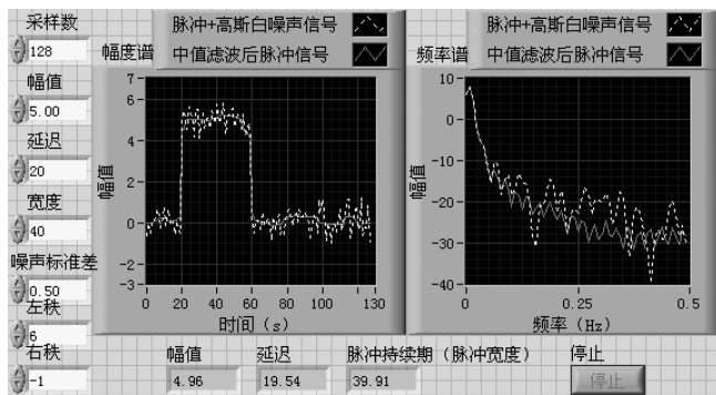
图 5-43 使用中值滤波器 VI 对混有高斯白噪声的脉冲信号进行滤波
