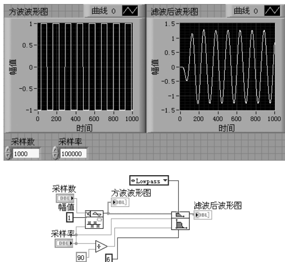
图 5-30 巴特沃斯低通滤波器对采集的方波信号滤波
