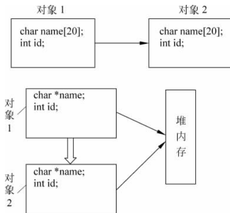
图 3.1 浅拷贝的两种情况
