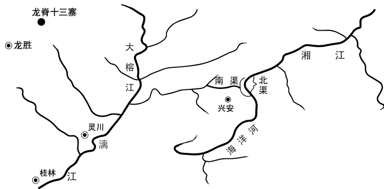
灵渠位置示意图：灵渠分为南渠和北渠，打通了湘江和漓江之间的水运，将长江水系和珠江水系连通起来
