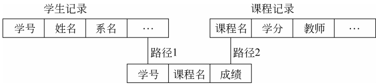
图 5.1 学生选课管理中的数据联系
