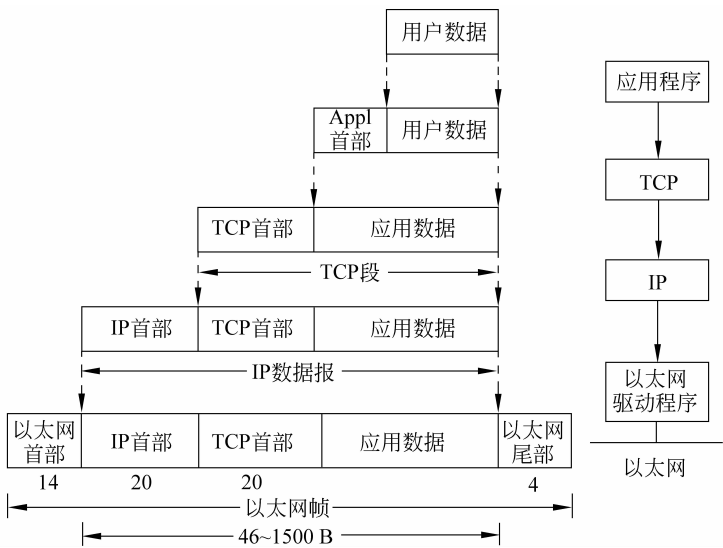
图 3.1.1 TCP/IP 协议系统
