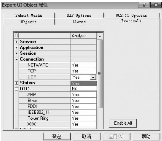
图 3.2.19 指定分析协议设置
