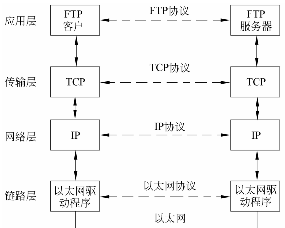
图 3.1.2 逻辑通信结构
