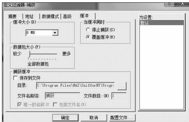
图 3.2.16 捕获缓冲区设置
