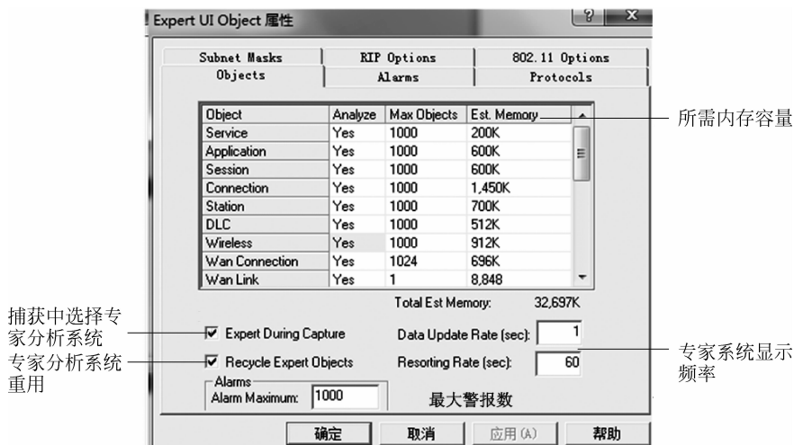
图 3.2.17 专家选项设置
