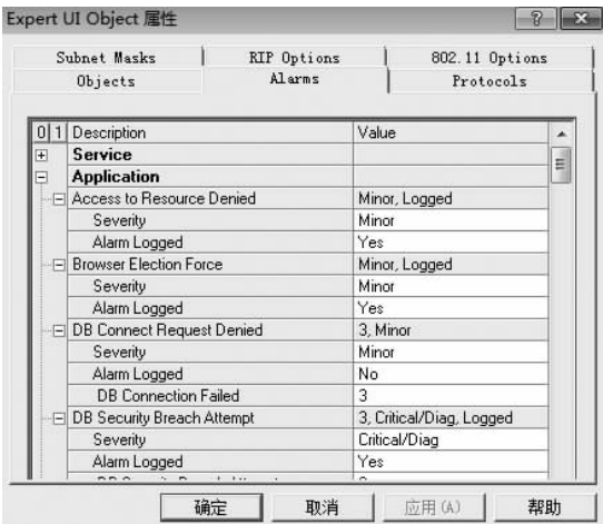
图 3.2.18 专家系统阈值设置
