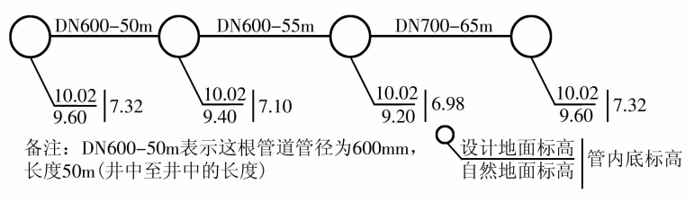
图 1-1 管道布置示意图
