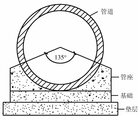
图 1-2 基础断面示意图
