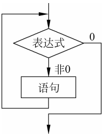
图 3-4 当循环结构
