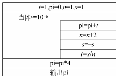
图 3-9 N-S 流程图
