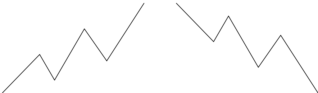
图 3.2 上升趋势
