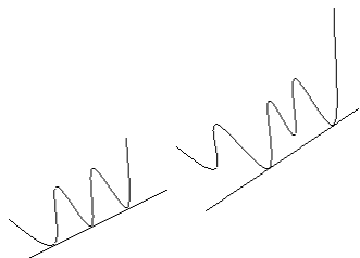
图 3.10 上升支撑线
