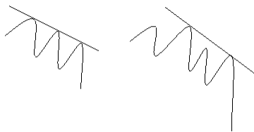
图 3.11 下降压力线
