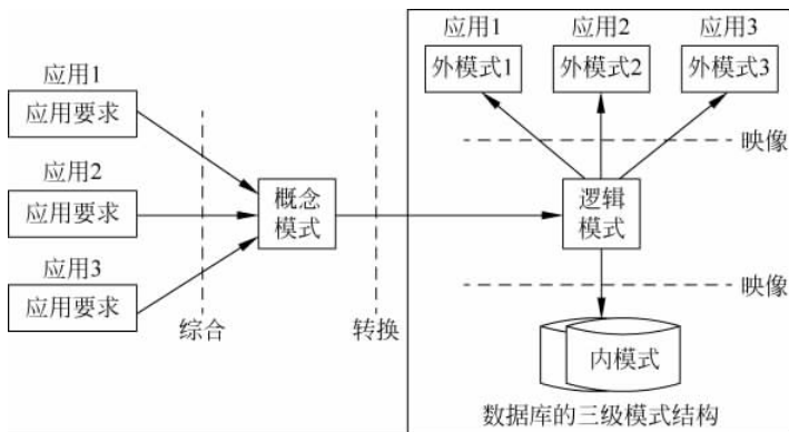
图 3-2 数据库的各级模式
