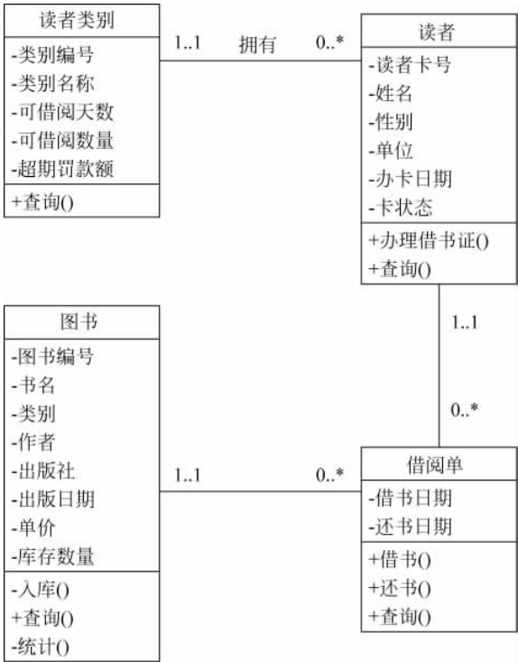
图 3-13 高校图书管理系统类图
