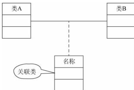
图 3-8 关联类的表示示意图
