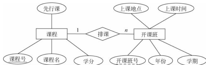
图 3-28 开课班弱实体集依赖于课程实体集
