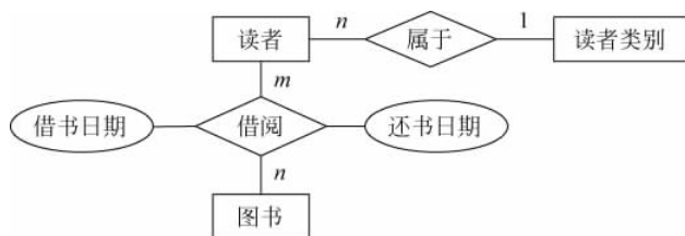
图 3-27 高校图书管理系统实体联系图
