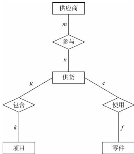
图 3-34 多元联系转换为等价的二元联系
