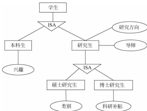
图 3-32 学生实体的层次关系
