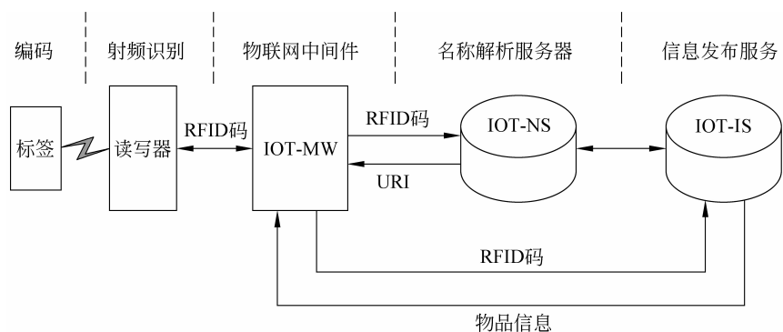
图 5.6 物联网（IOT）EPC 网络结构示意图
