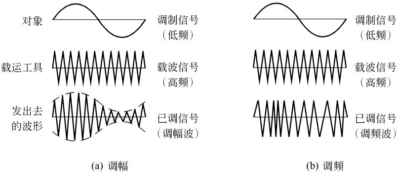
图 1-3 调制的波形
