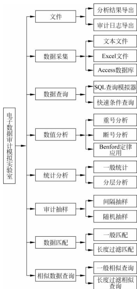
图 3.5 “电子数据审计模拟实验室”软件 V1.0 的主要功能
