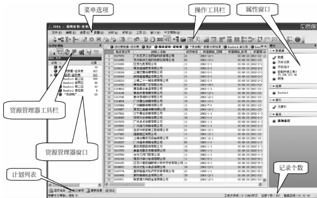
图 3.8 IDEA 8 的主界面
