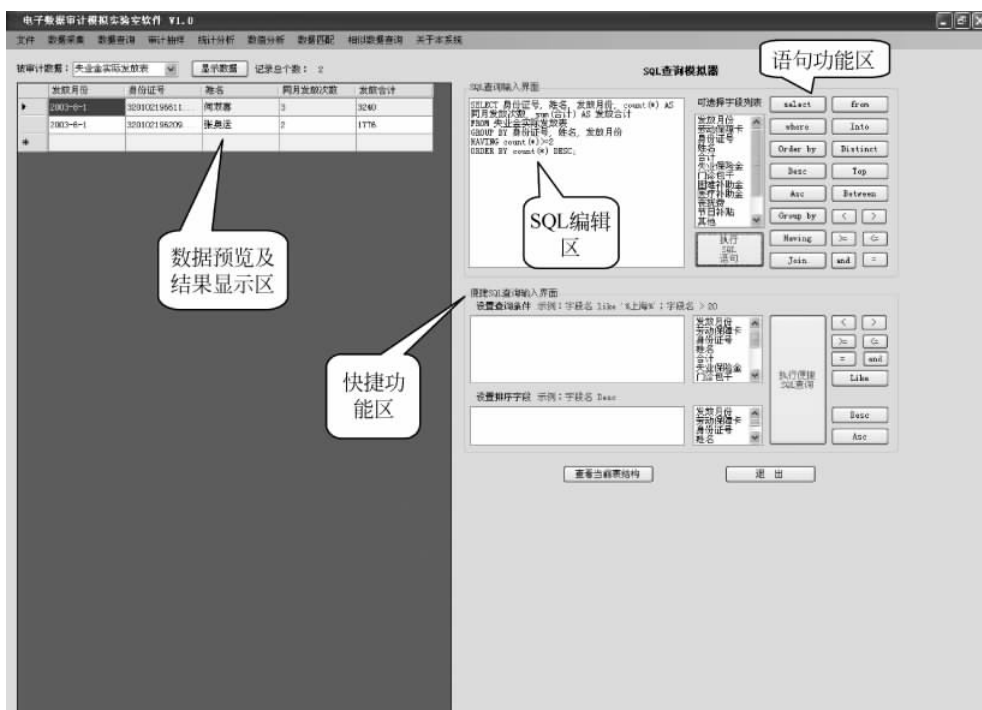
图 3.7 “电子数据审计模拟实验室软件 V1.0”的 SQL 查询模拟器功能主界面
