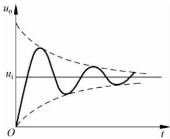
图 3.1-14 振荡环节的阶跃响应
