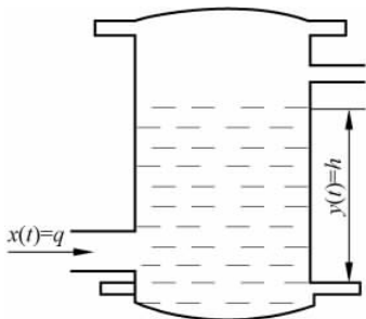
图 3.1-10 积分环节示意图
