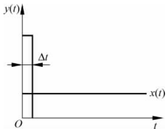
图 3.1-12 微分环节的阶跃响应
