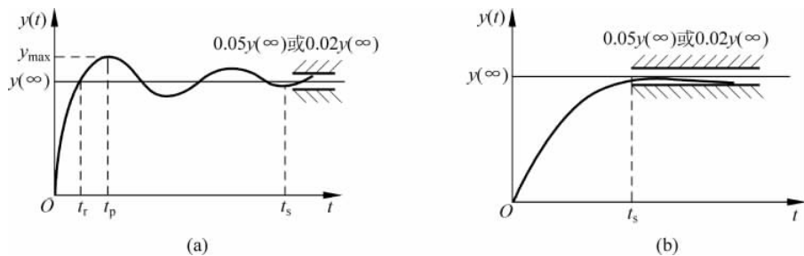
图 3.1-21 稳定系统的阶跃响应曲线
