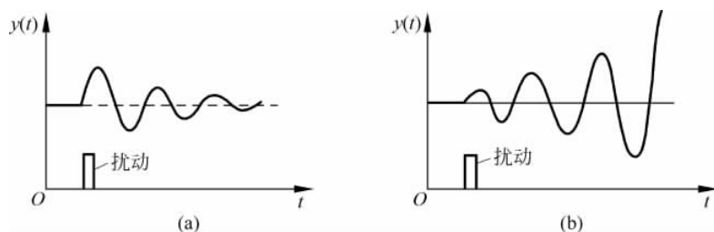
图 3.1-18 稳定与不稳定系统
