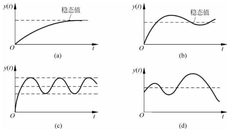
图 3.1-20 自动控制系统的动态过程
