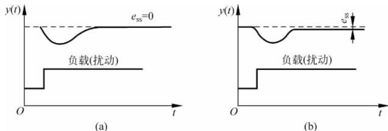
图 3.1-19 有静差与无静差系统
