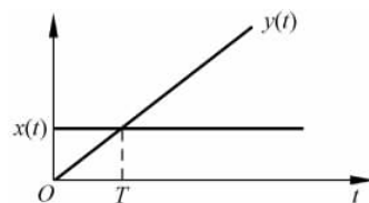
图 3.1-11 积分环节的阶跃响应
