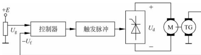
图 3.1-6 闭环控制系统原理图
