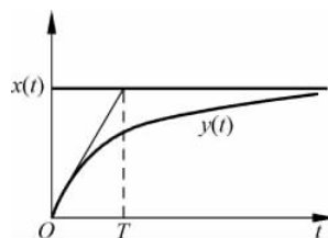
图 3.1-9 惯性环节的阶跃响应
