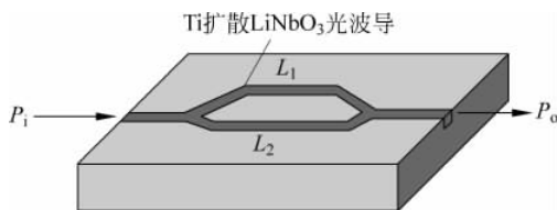
图 3-28 \text{LiNbO}_3 光波导温度传感器结构示意图
