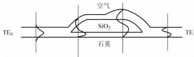
图 3-20 分支光波导模变换器
