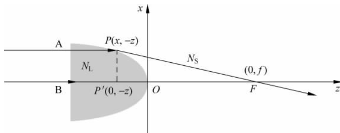
图 3-21 模折射率透镜示意图
