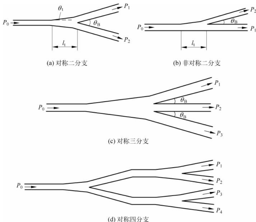
图 3-7 对称和非对称分支光波导
