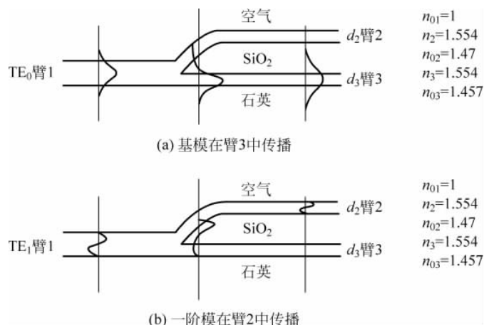
图 3-18 三层结构分支光波导
