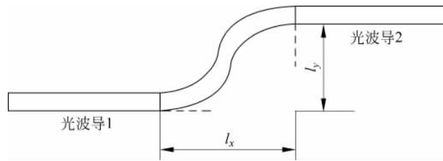
图 3-6 曲率渐变连接
