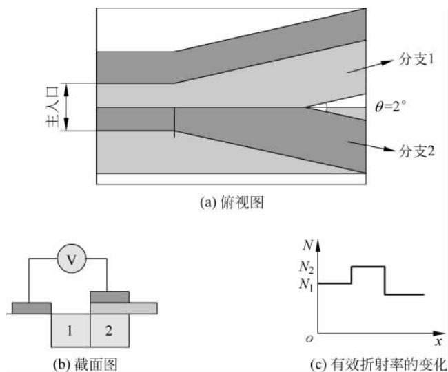
图 3-19 Y 形分支光波导模分割器
