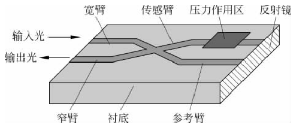
图 3-29 光波导压力传感器结构示意图
