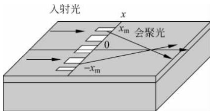
图 3-25 折射率分布型
