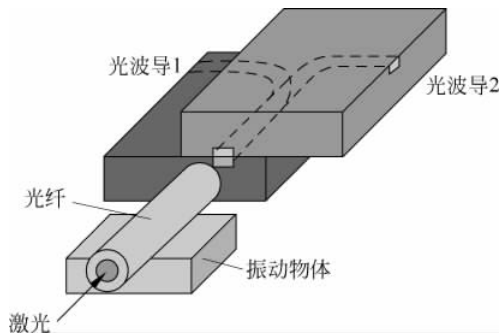
图 3-31 振动传感器结构示意图
