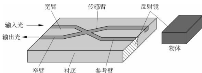
图 3-30 微位移传感器结构示意图
