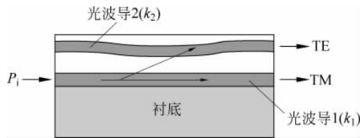
图 3-17 方向耦合器型模分割器
