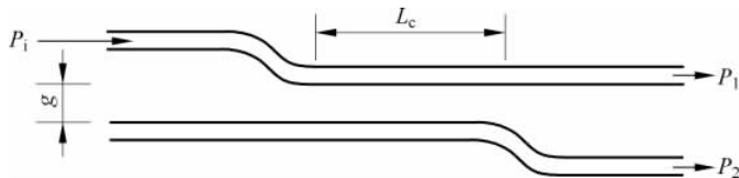
图 3-8 双通道方向耦合器
