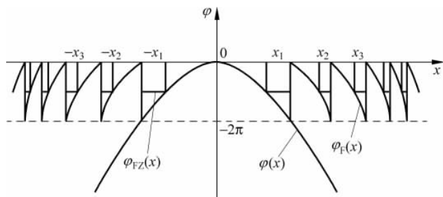
图 3-24 利用费涅耳透镜进行的位相调制
