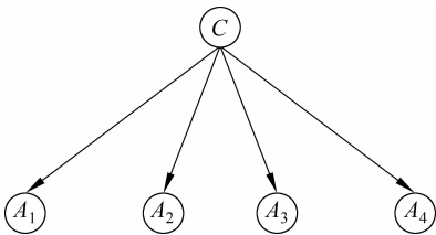
图 5-4 朴素贝叶斯分类器的结构
