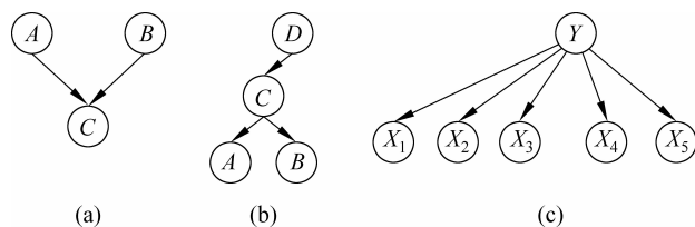
图 5-2 贝叶斯信念网络
