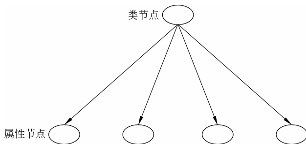
图 5-1 朴素贝叶斯分类器的结构示意图
