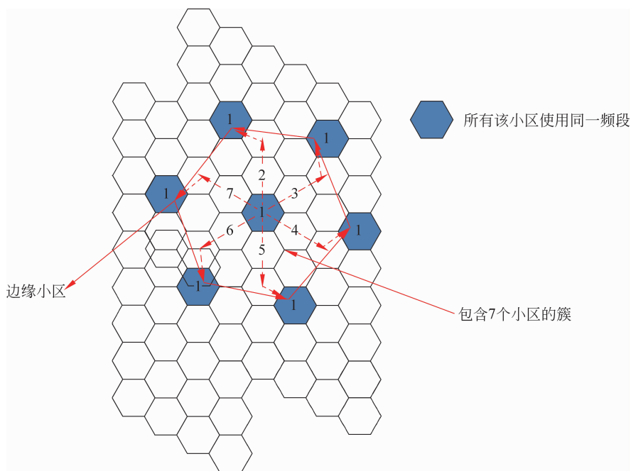
图 3-1 蜂窝通信系统
