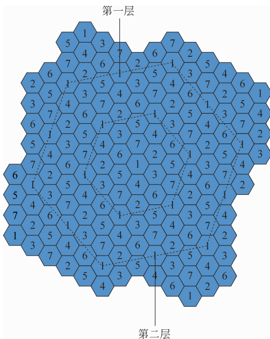
图 3-5 N=7 时的两层同信道干扰小区
