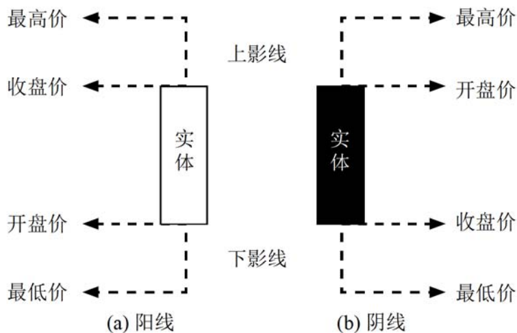
图1.2 阳线和阴线
