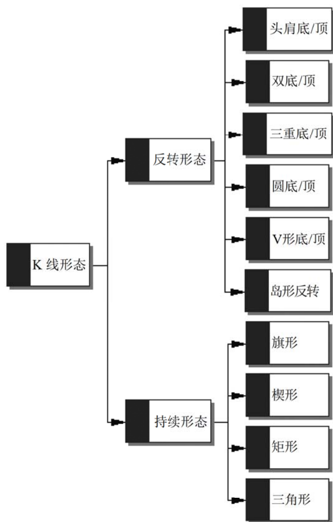
图1.19 K线形态
