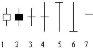
图1.16 无势K线
