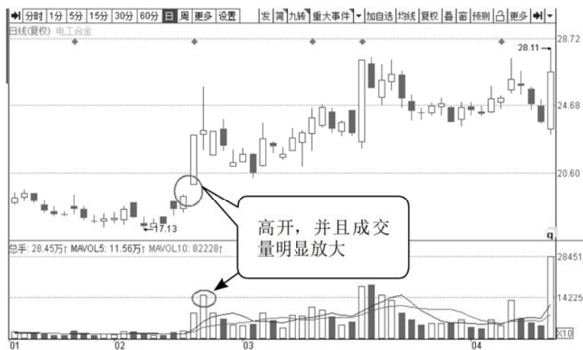
图1.3 高开
