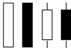
图1.13 强势K线
