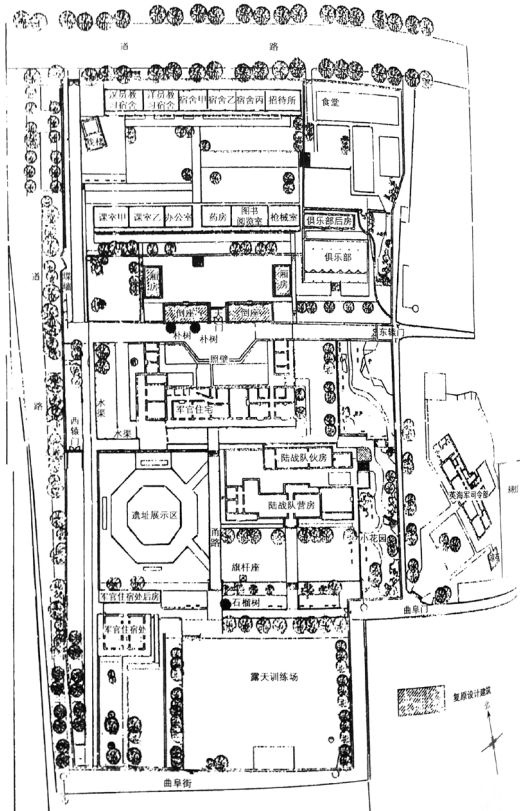
威海水师学堂总平面图
