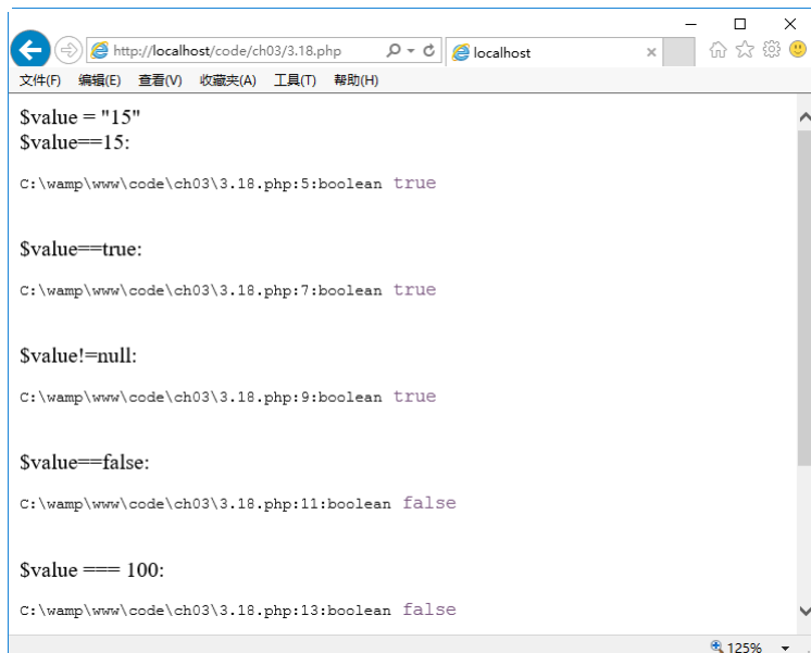
图 2-20 使用比较运算符
