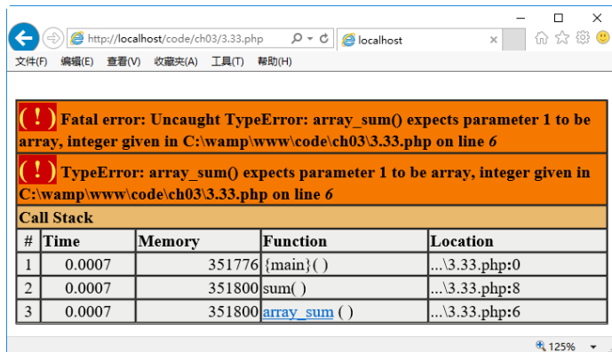
图 2-16 错误提示信息
