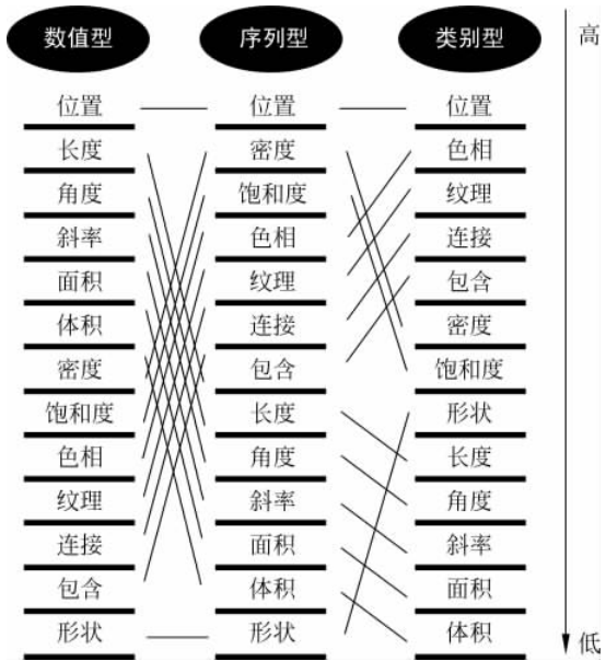
图 3-12 视觉通道在不同数据可视化编码的优先级
