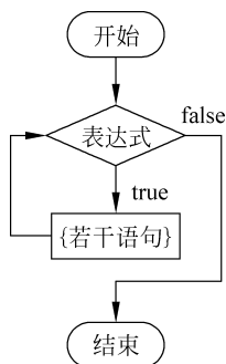
图 3.8 while 循环语句
