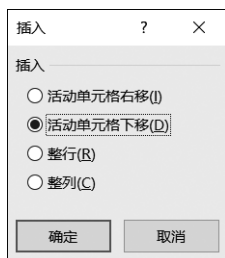
图 5-13 “插入”对话框
