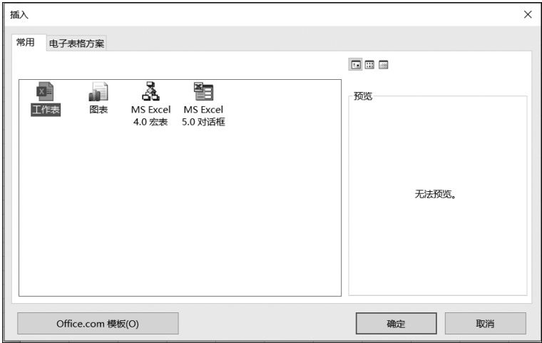
图 5-10 “插入”对话框
