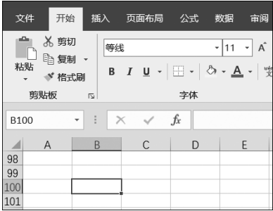
图 5-12 活动单元格
