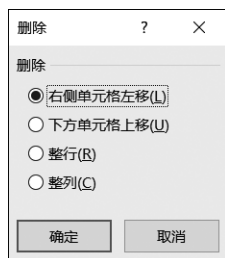
图 5-14 “删除”对话框
