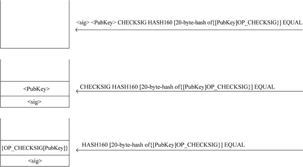
图 3-27 < sig > PubKey >和操作符 CHECKSIG 入栈示意图
