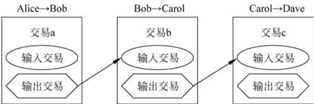
图 3-19 一系列单输入/单输出交易示意图
