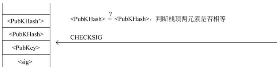
图 3-25 OP_EQUALVERIFY 操作示意图
