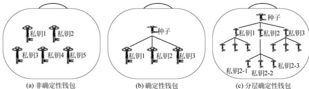
图 3-18 三种数字钱包示意图
