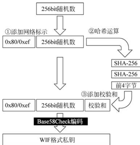
图 3-16 WIF 格式私钥产生过程示意图
