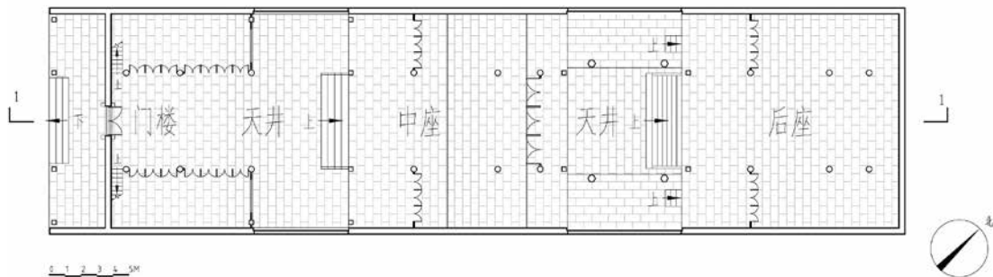
图1 新会书院平面图
