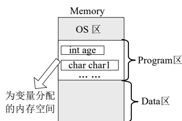
图 3.2 变量占用的内存空间
