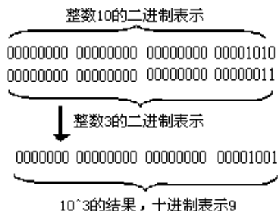
图 3.8 10 ^ 3 的运算过程
