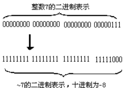
图 3.7 ~7 的运算过程
