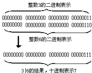
图 3.6 3 | 6 的运算过程
