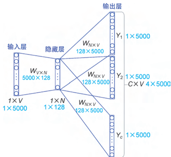
图 5.16 Skip-gram 算法实现
