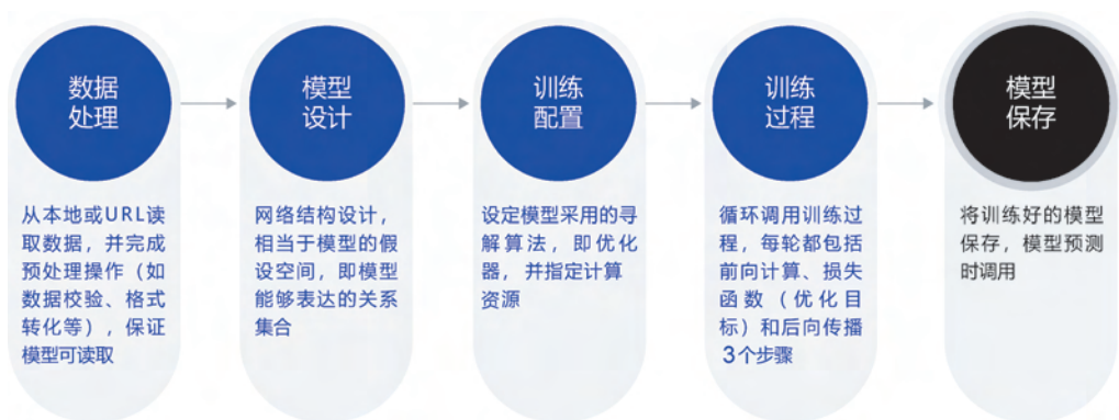
图 5.10 使用飞桨框架构建神经网络过程
