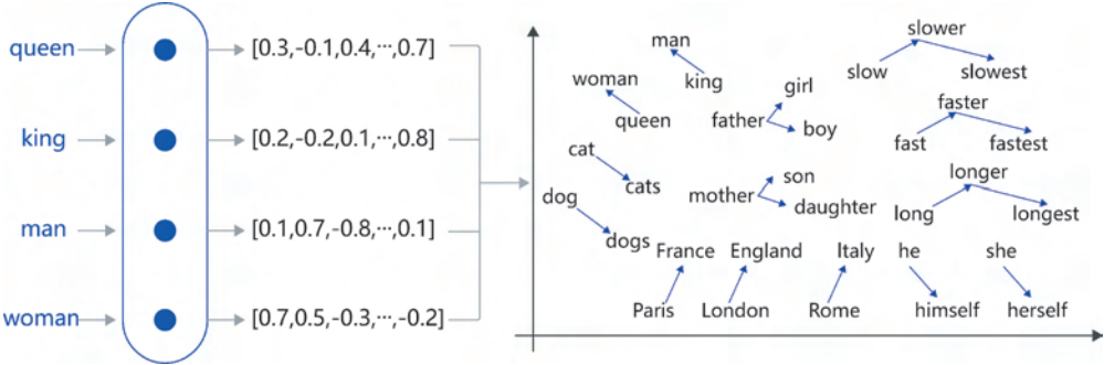
图 5.11 词嵌入计算示意图
