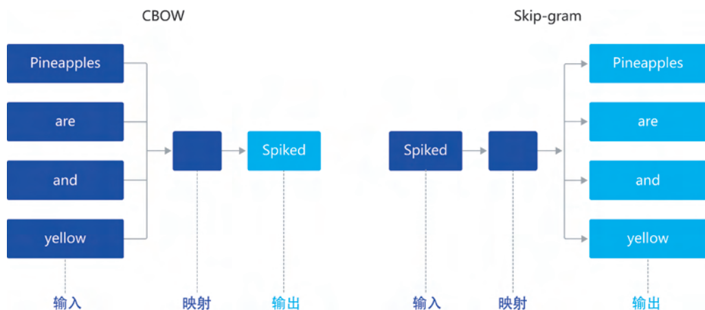
图 5.14 CBOW 和 Skip-gram 语义学习示意图
