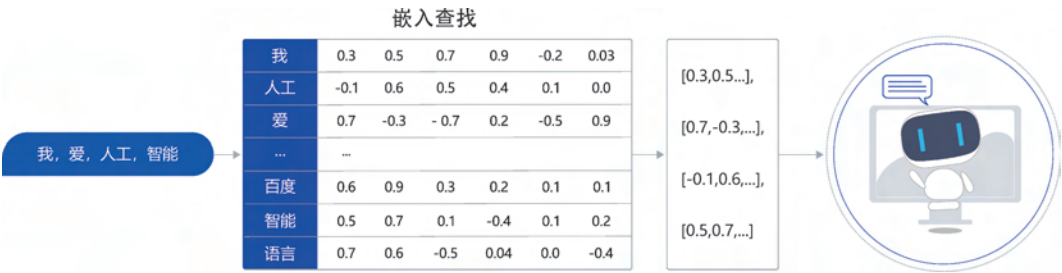
图 5.12 词嵌入查询表
