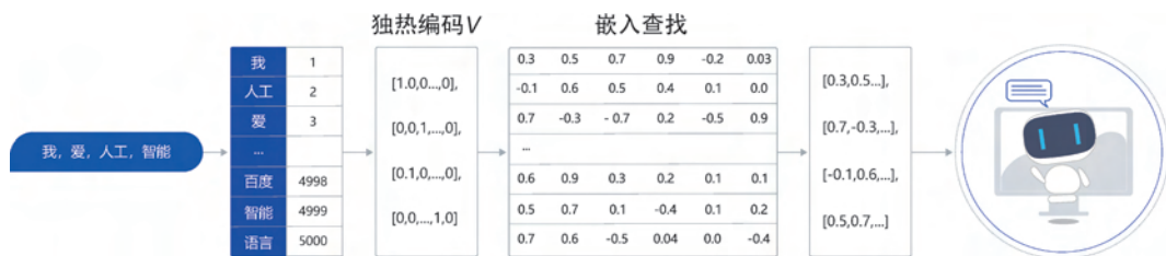
图 5.13 张量计算示意图
