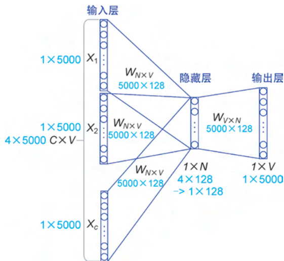
图 5.15 CBOW 的算法实现
