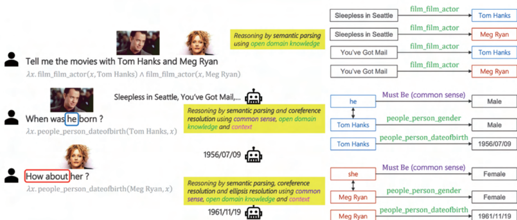
图 5.7 多轮对话中的指代和省略
