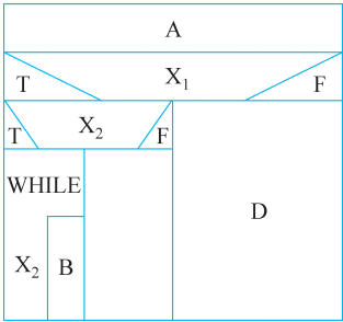
图 5-13 N-S 图示例
