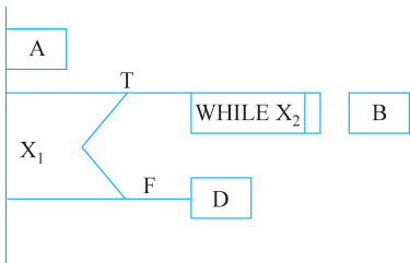
图 5-18 PAD 示例
