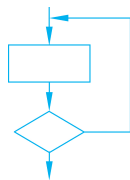
图 5-4 UNTIL 型循环
