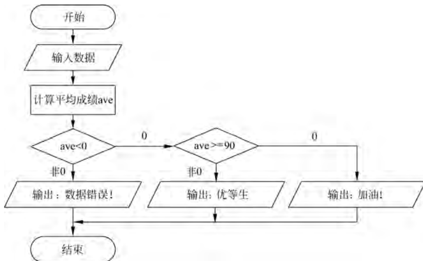
图 3-7 if 命令的嵌套结构示例
