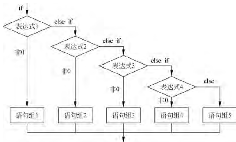
图 3-8 if-else if 结构的流程图
