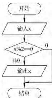
图 3-13 编程题 1 的算法流程图
