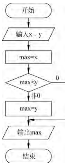
图 3-14 编程题 2 的算法流程图
