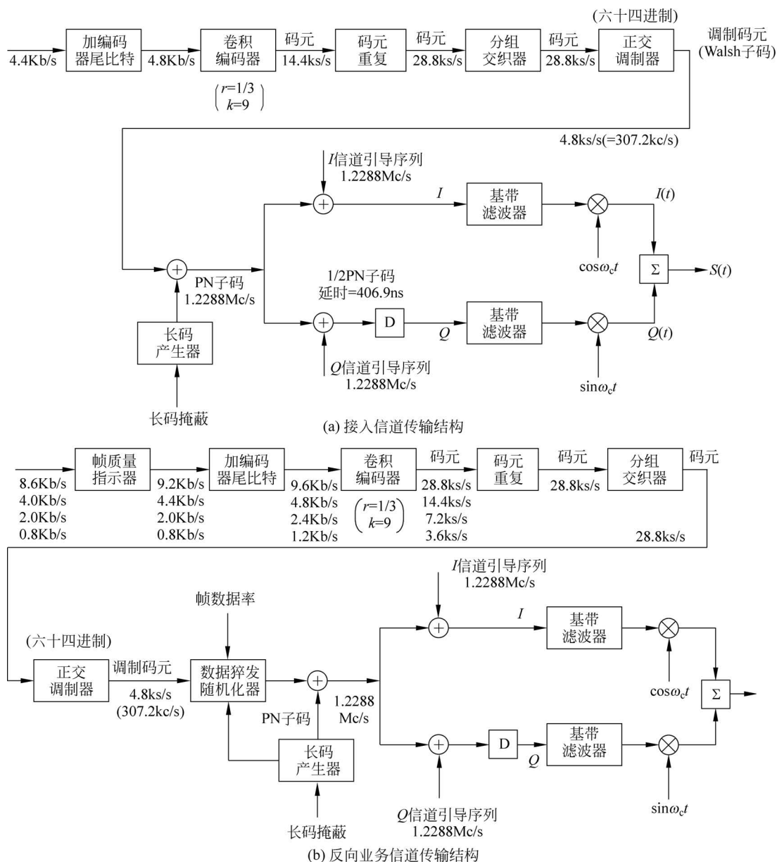
图 3-26 IS-95 CDMA 反向信道传输的结构
