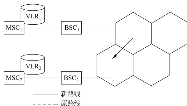
图 3-20 不同 MSC/VLR 控制的小区之间的切换过程
