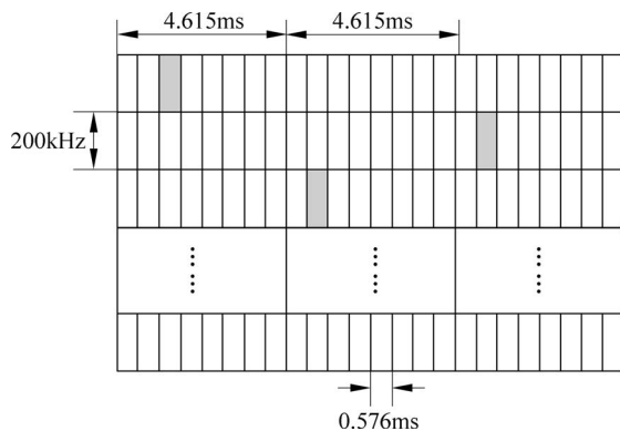
图 3-17 GSM 跳频示意图
