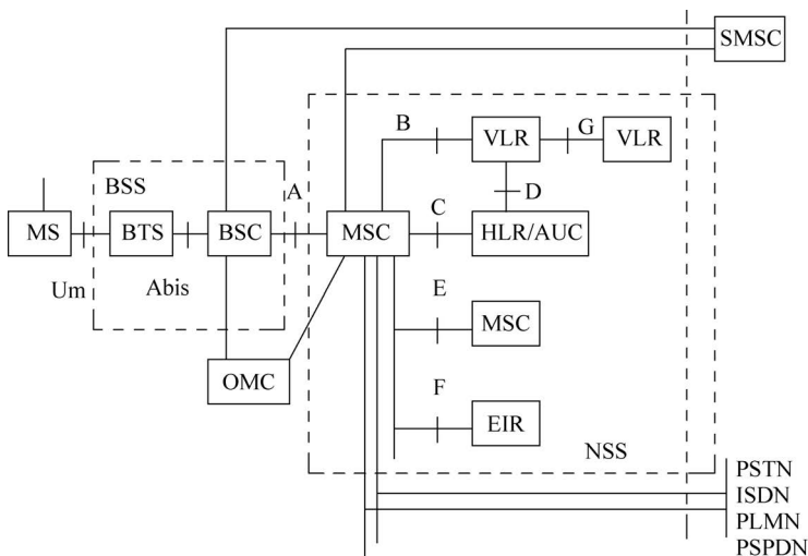
图 3-1 GSM 网络结构
