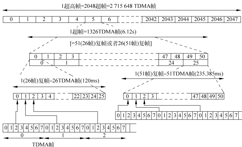
图 3-10 GSM 的各种帧结构
