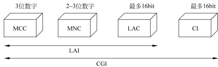
图 3-7 CGI 的格式
