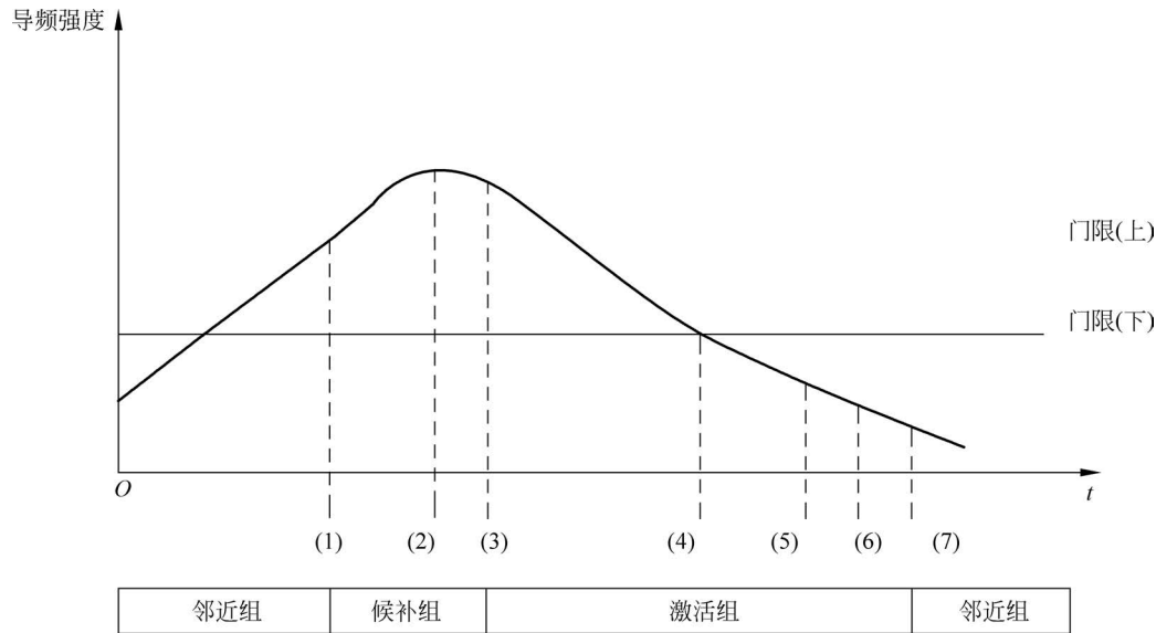
图 3-27 软切换过程
