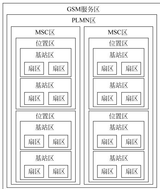
图 3-2 GSM 服务区域划分
