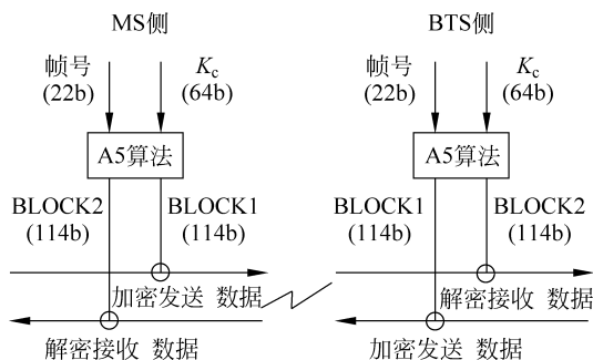
图 3-22 GSM 加密模式传输过程
