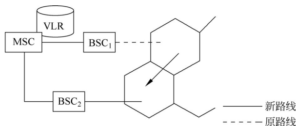
图 3-19 同一 MSC/VLR 内不同 BSC 控制小区之间的切换过程
