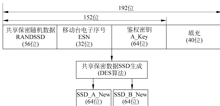
图 3-28 SSD 产生过程
