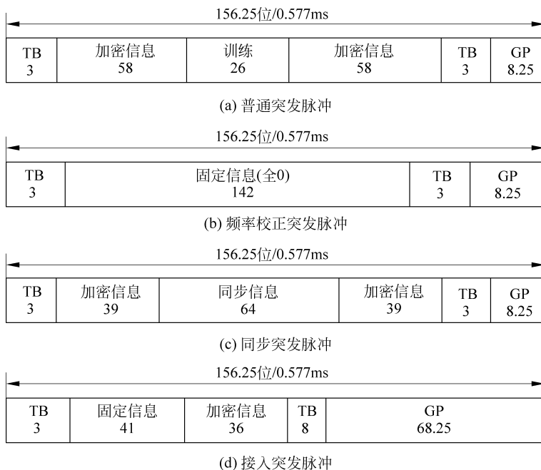
图 3-11 4 种不同功能突发脉冲序列的格式
