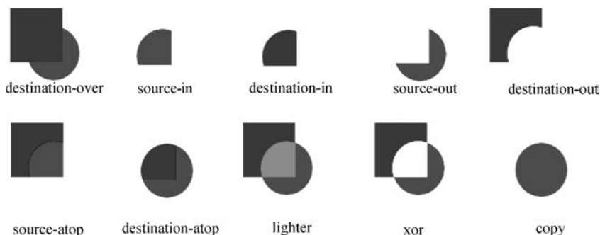
图 5-9 globalCompositeOperation 属性的不同取值效果
