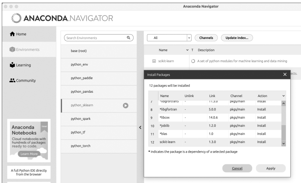
图 5.4 在虚拟环境 python_sklearn 中使用 Anaconda Navigator 搭建和配置 Scikit-learn
