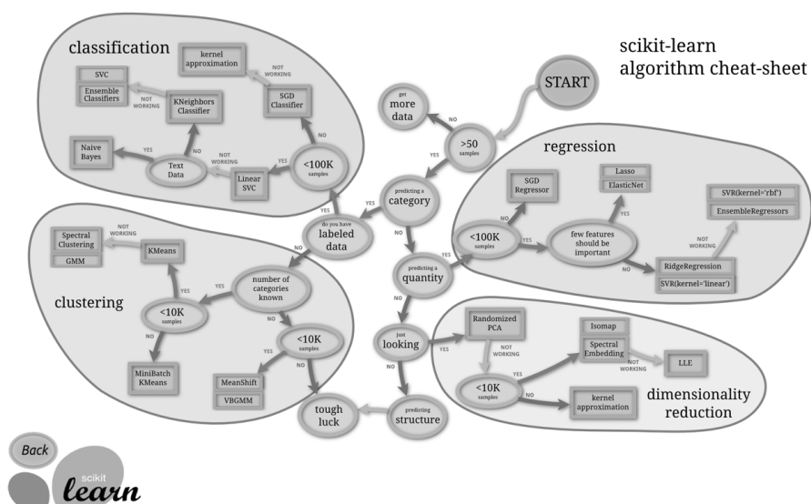
图 5.1 Scikit-learn 主要机器学习模型的全景图
