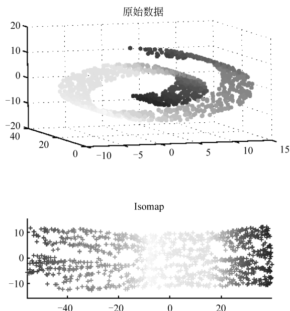
图 5.8 Isomap 解决了 3D 流形分布数据的 2D 降维问题
