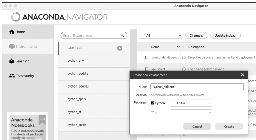
图 5.2 使用 Anaconda Navigator 创建用于单机机器学习的虚拟环境 python_sklearn
