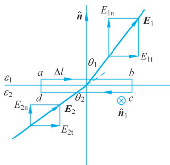
图 5.6 E 切向分量的边界条件
