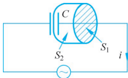
图 5.4 安培环路定律应用于时变场时出现的矛盾
