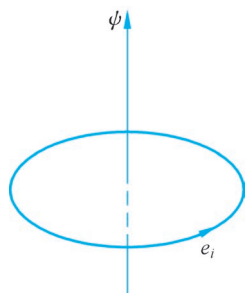
图 5.1 e_i 和 \psi 的正方向 满足右手法则
