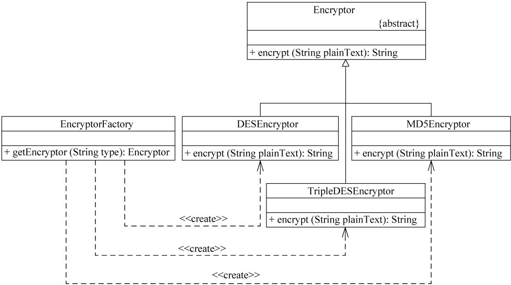
图 3-3 加密算法库结构图
