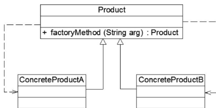
图 3-6 简化的简单工厂模式
