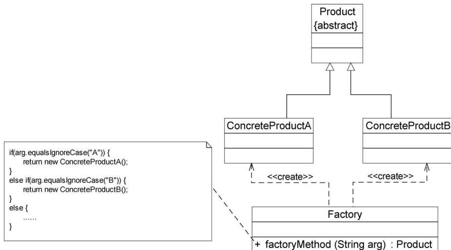
图 3-2 简单工厂模式结构图
