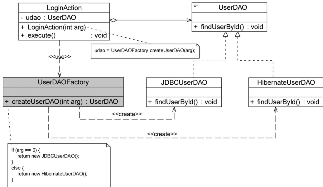
图 3-4 引入工厂类之后的结构图
