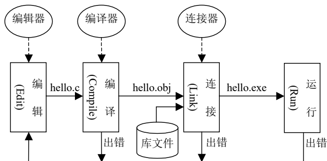
图 1.6 运行 C 程序的步骤
