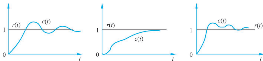
图 3-24 高阶系统的单位阶跃响应曲线
