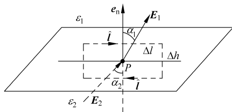
图 5-2 切向电场边界条件问题
