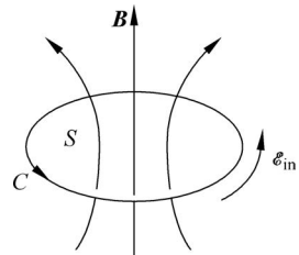
图 5-1 感应电动势与磁通变化的关系
