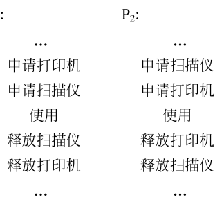
图 5-5 死锁状态示意图
