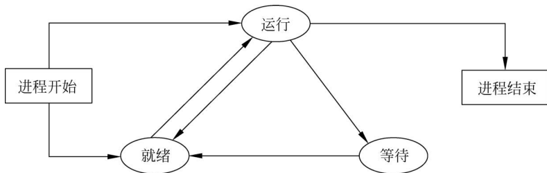
图 5-3 进程状态转换
