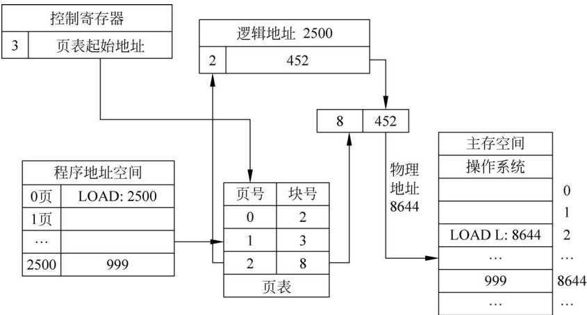
图 5-9 分页存储管理页表及地址转换示意图
