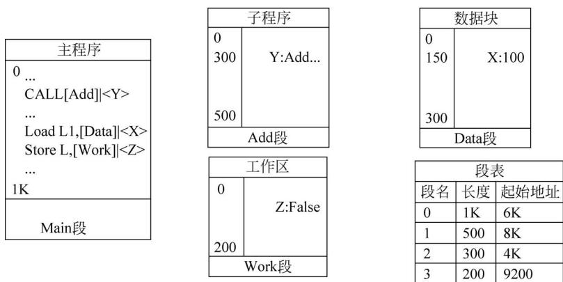
图 5-12 分段地址空间示意图
