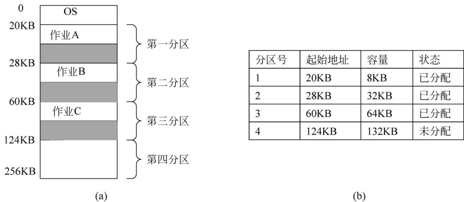
图 5-8 固定分区管理示意图
