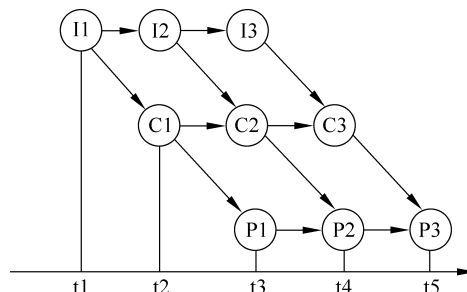
图 5-2 多道程序并发执行示意图
