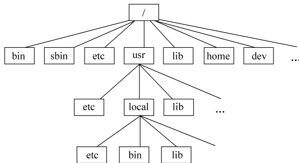
图 5-15 树状目录结构
