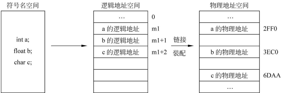
图 5-7 静态地址重定位示意图
