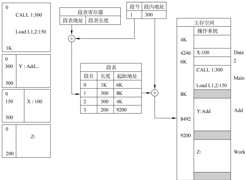
图 5-13 分段存储管理地址转换示意图
