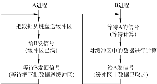
图 5-4 进程同步示意图
