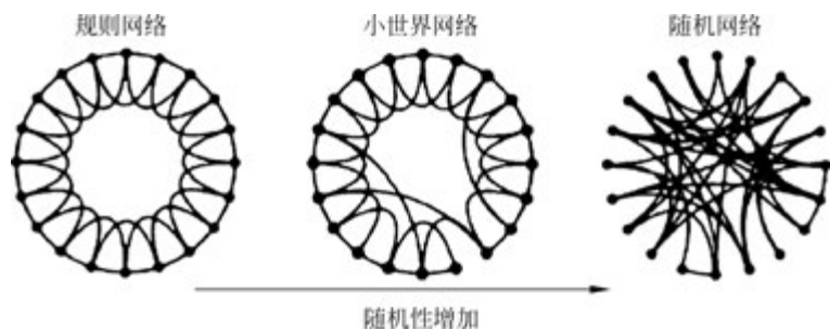
图 3-4 规则网络、小世界网络与随机网络示意图
