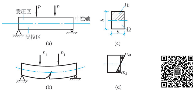
图 1-2 素混凝土结构
