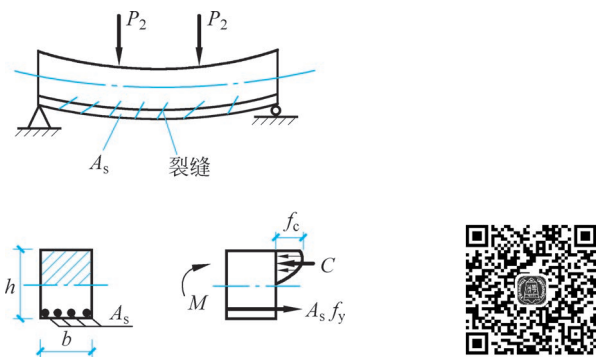
图 1-3 钢筋混凝土结构
