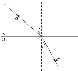
图 1-4 光线的折射
