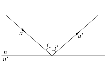
图 1-3 光线的反射
