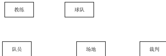
图 3-1 实体联系图
