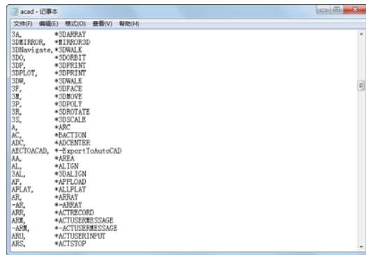
图 1-27 acad-记事本中的简写命令
