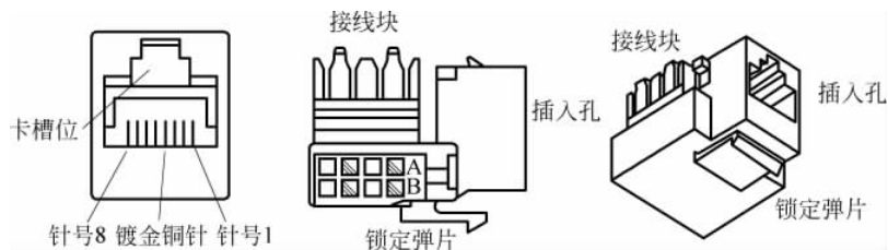
图 3-22 模块正视图、侧视图、立体图
