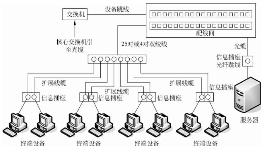
图 3-16 区域布线示例
