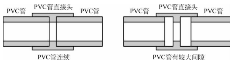
图 3-29 PVC 管连接示意图
