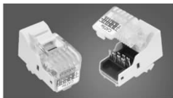
图 3-25 免打线工具模块
