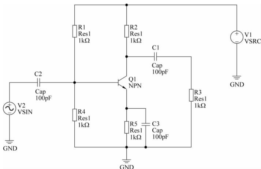
图 3-81 为电路元器件和信号源分配唯一的标识符
