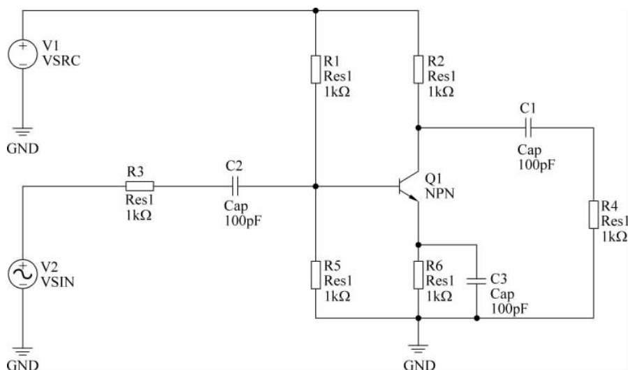
图 3-51 为电路元件和信号源分配唯一的标识符
