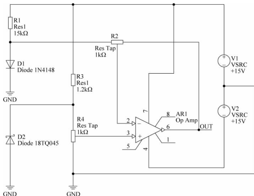
图 3-75 修改电路元件参数
