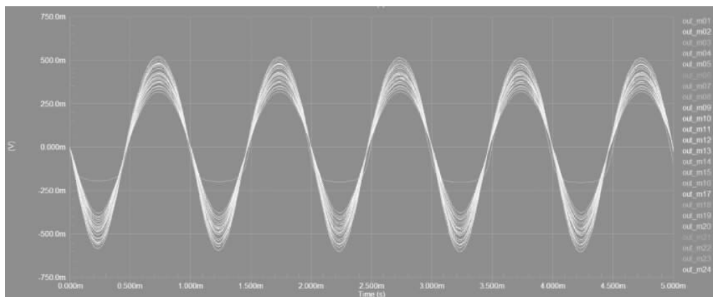
图 3-86 蒙特卡罗分析结果
