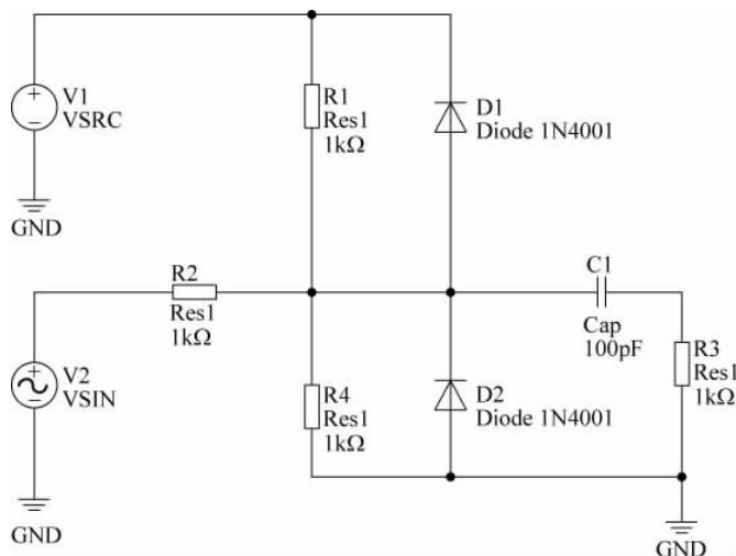
图 3-25 为电路中的元器件分配唯一的标识符
