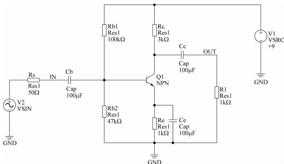
题图 晶体管小信号放大电路
