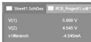
图 3-14 计算电流的结果
