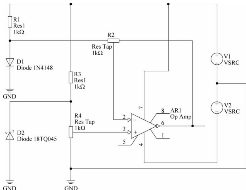
图 3-74 为电路元器件和信号源分配唯一的标识
