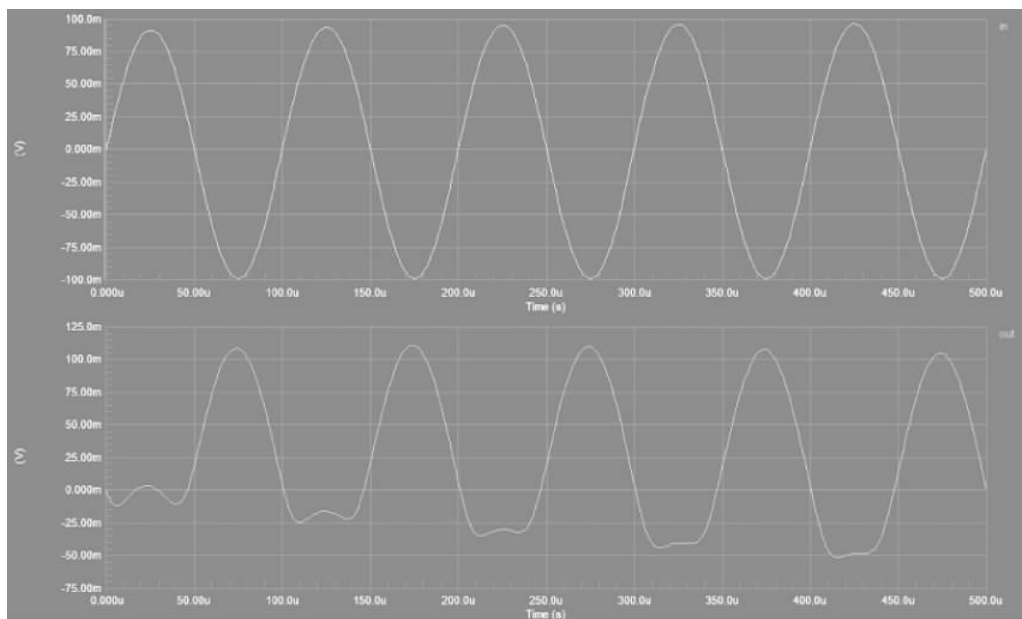
图 3-60 瞬态分析结果
