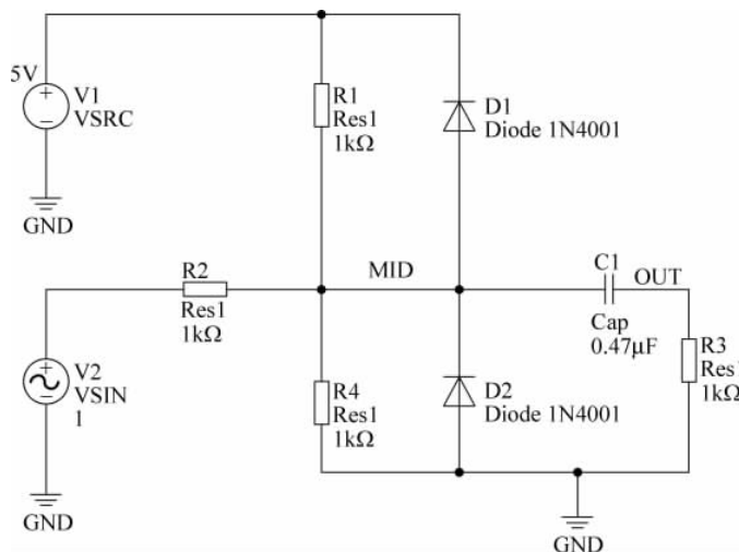
图 3-29 为电路指定网络标识符
