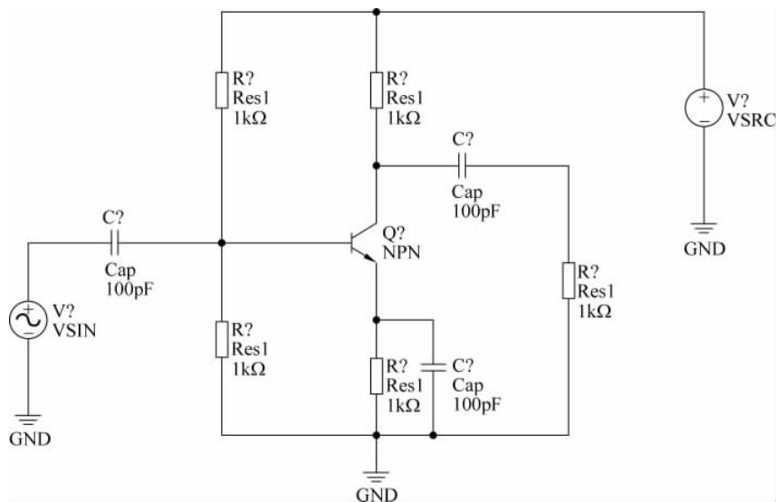
图 3-80 连接电路元器件和信号源
