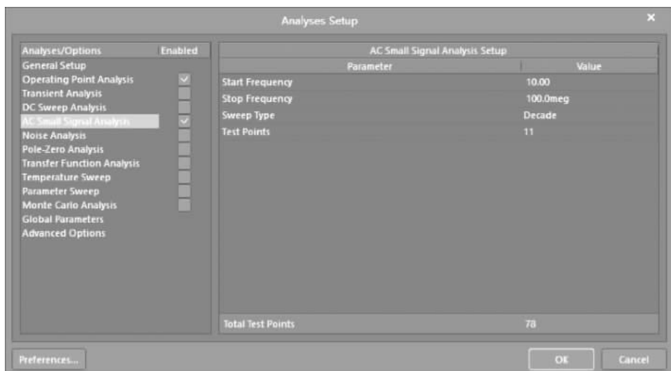
图 3-31 设置交流分析参数
