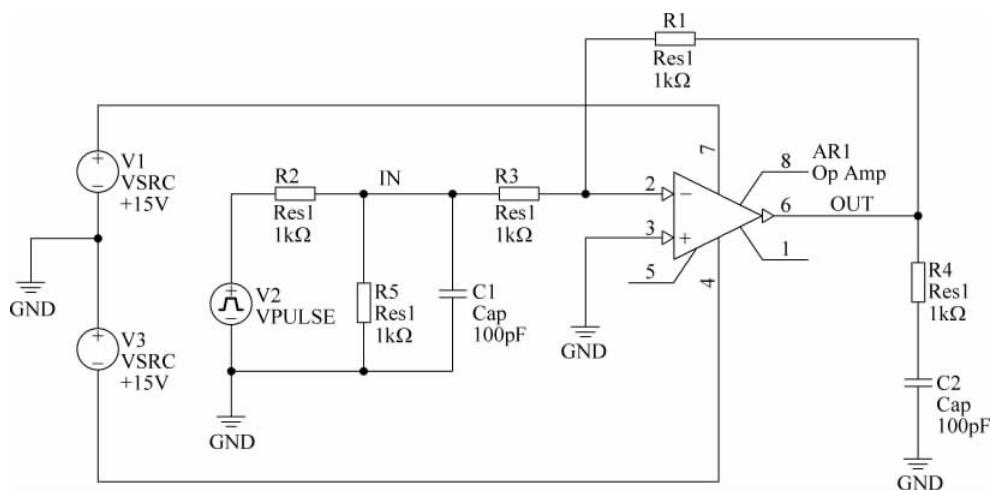
图 3-40 添加 IN 和 OUT 网络标号
