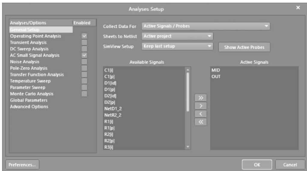
图 3-30 设置通用分析参数
