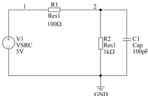
图 3-9 指定网络标号
