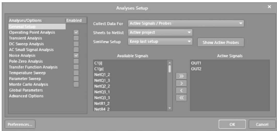
图 3-68 设置仿真参数界面 1
